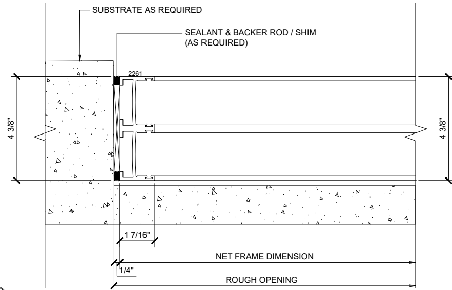
① JAMB MAX SLIDING DOORS (OXXO) SCALE: 6"=1'-0"
